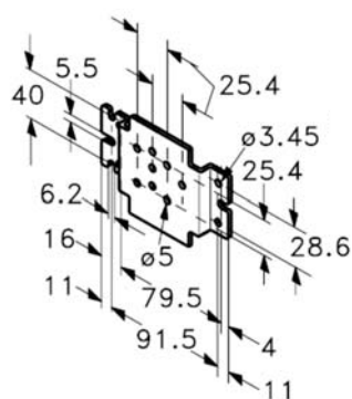
Nástěnná konzola
