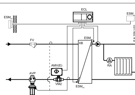
Nepriamo pripojený systém vykurovania
