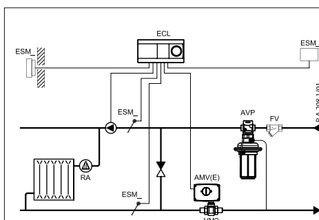
Priamo pripojený systém vykurovania
