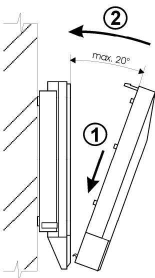
Obrázek 1: Montáž snímače
