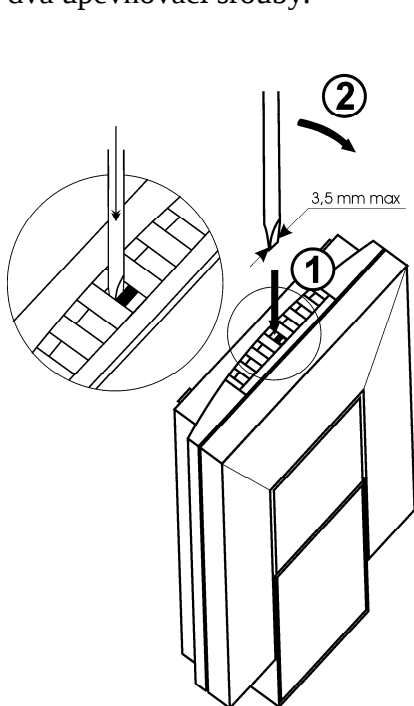
Obrázek 2: Demontáž snímače
